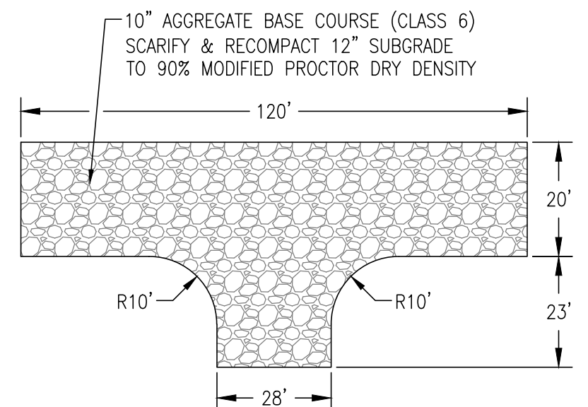
GRAVEL TURNAROUND N.T.S.
